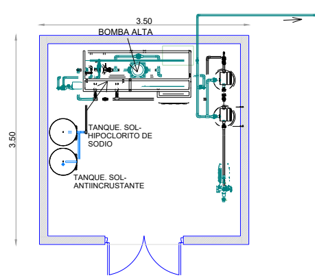
PLANTA CASETA PTAP
