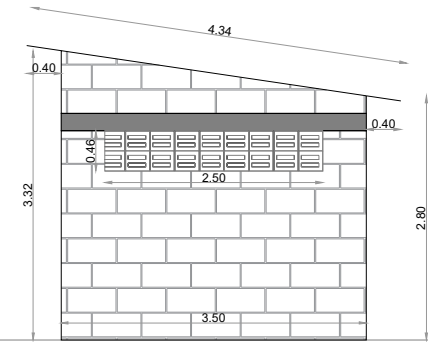
FACHADA LATERAL 2
