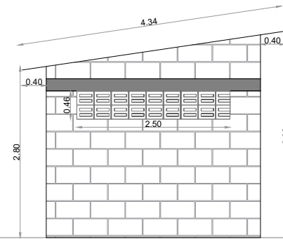
FACHADA LATERAL 1
