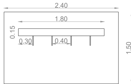
VISTA EN PLANTA PUNTO DE SUMINISTRO AGUA CRUDA
